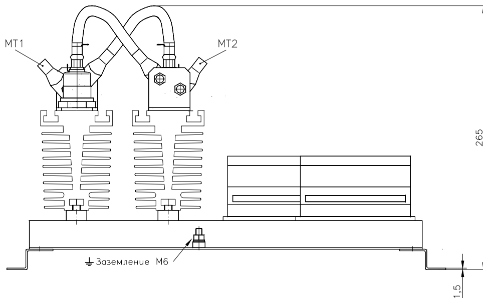
Рис. 1 – Внешний вид и габаритно-установочные размеры
