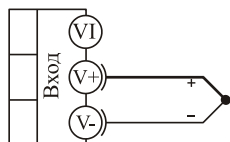
термопара
