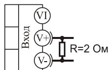
0...40 мА токовый выход
