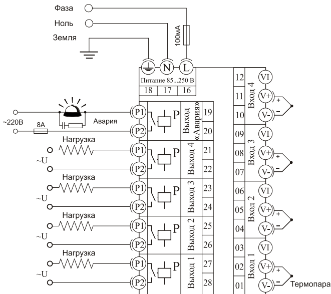
Рис 2. Типовая схема подключения Термодат-13К5 для регулирования температуры по четырем каналам
