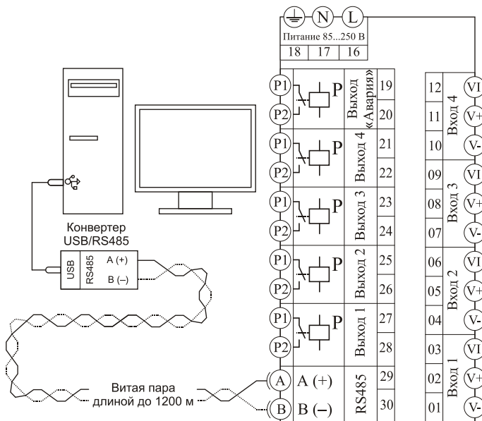
Рис 1. Подключение к компьютеру (для приборов с интерфейсом)
