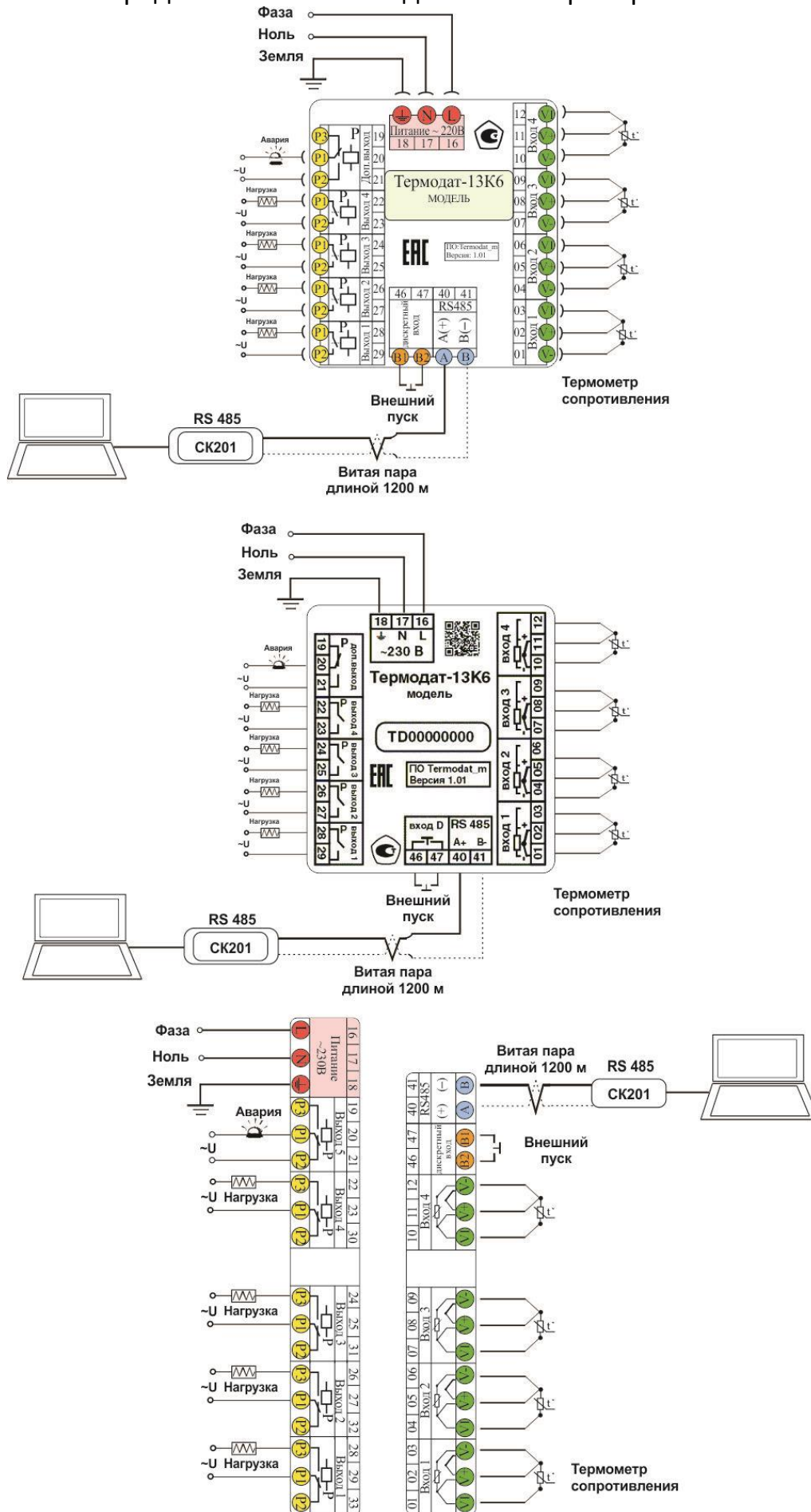
Рисунок 12 – Схема подключения прибора
