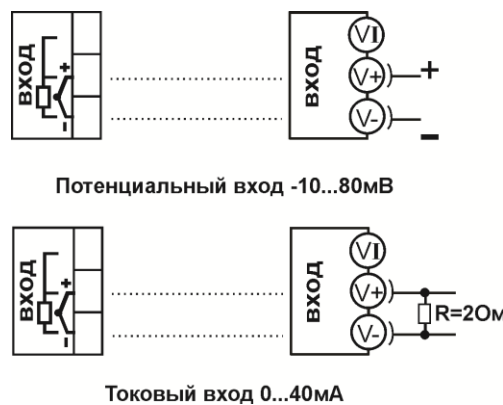
Рисунок 8 - схема подключения датчика с токовым выходом к входу прибора.
