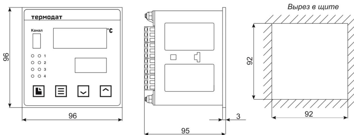
Рисунок 14 – Габаритные размеры прибора Термодат 13К6/.../
