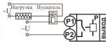
Подключение нагрузки мощностью до 2,3 кВт
