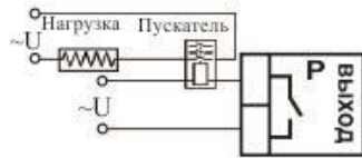
Подключение нагрузки мощностью до 2,3 кВт
