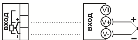
Рисунок 6 - Схема подключения термопары к входу прибора.
