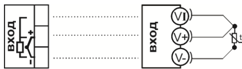
Рисунок 7 - Схема подключения термометра сопротивления к входу прибора
