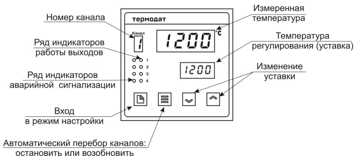
Рисунок 3 – Описание индикаторов и кнопок управления прибора Термодат-13К6/...
