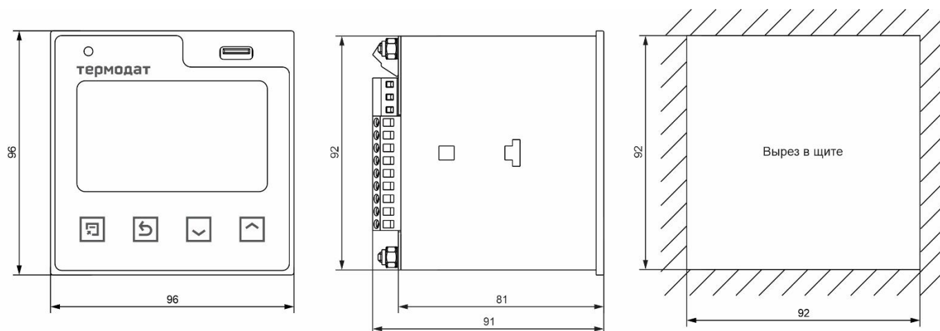
Рисунок 13 – Габаритные размеры прибора Термодат-16E6-A-(F)-(Eth)
