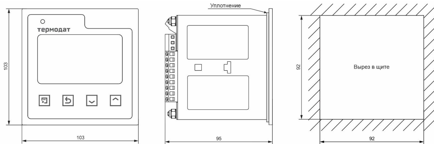
Рисунок 14 – Габаритные размеры прибора Термодат-16Е6-А7
