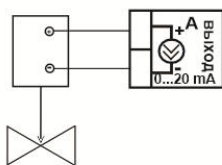
Подключение задвижки с электроприводом
