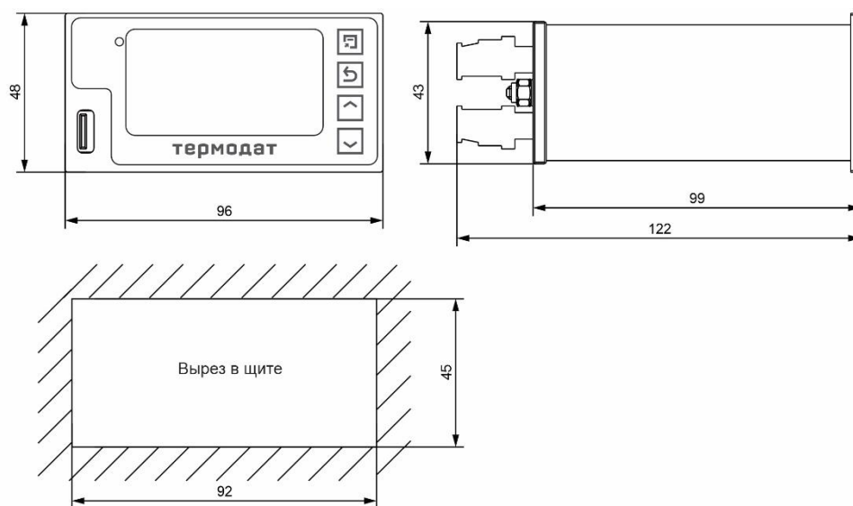
Рисунок 16 – Габаритные размеры прибора Термодат-16Е6-Н-(F)-(Eth)
