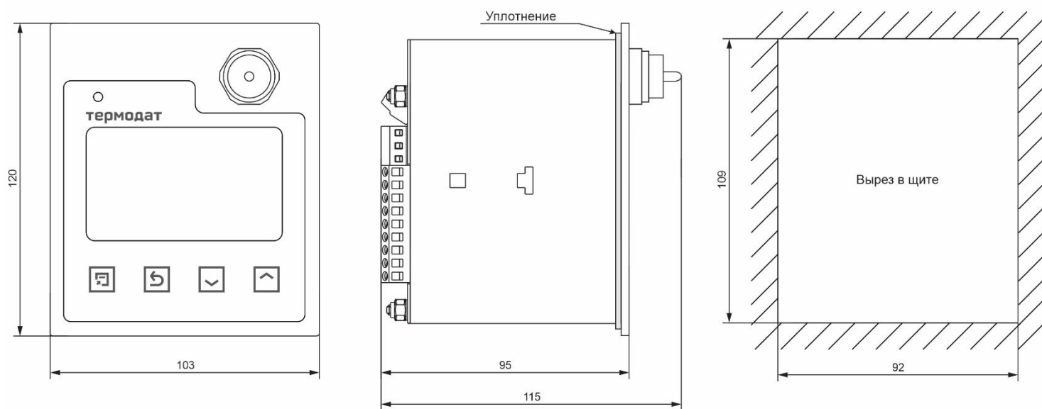
Рисунок 15 – Габаритные размеры прибора Термодат-16Е6-А9-Е
