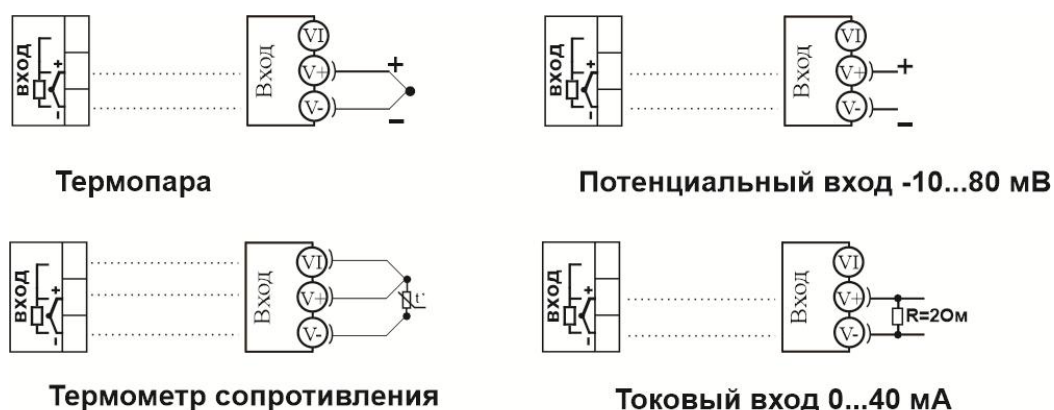
Рисунок 7 – Схемы подключения датчиков
