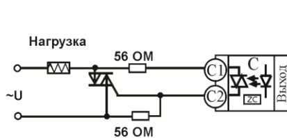
Подключение внешнего симистора
