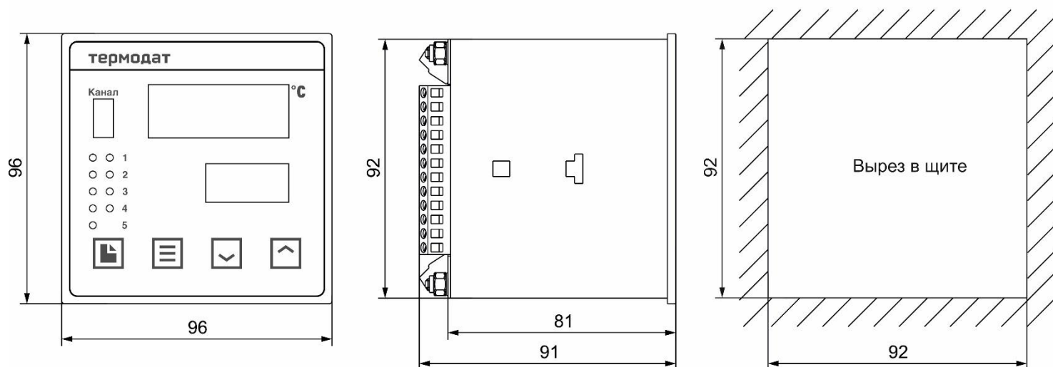
Рисунок 12 – Габаритные размеры прибора Термодат 13K6/.../
