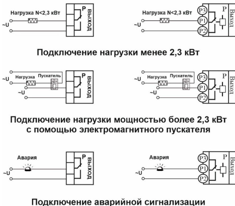
Рисунок 8 – Схемы подключения релейных выходов
