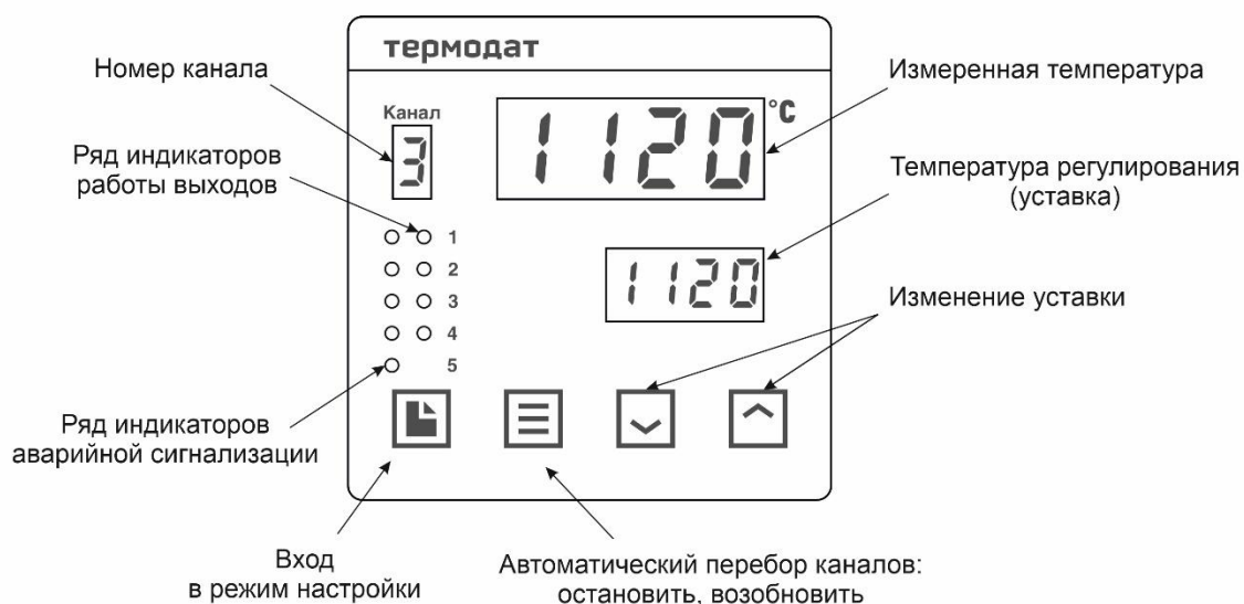
Рисунок 3 – Описание индикаторов и кнопок управления прибора Термодат-13К6/...
