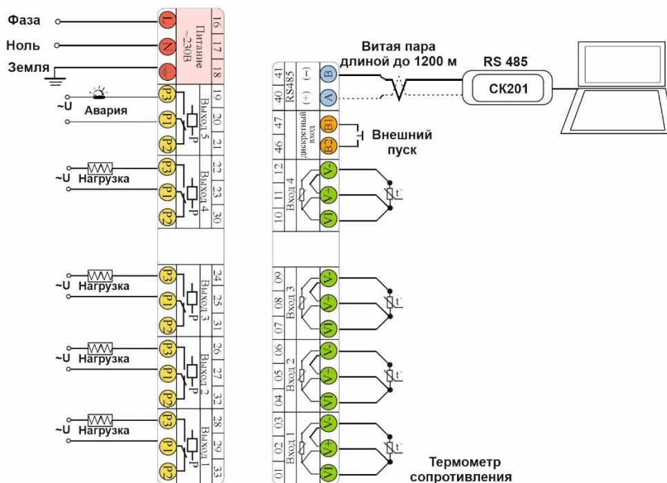
Рисунок 10 – Схема подключения прибора
