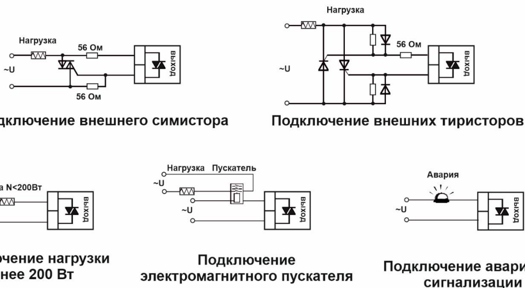
Рисунок 7 – Схемы подключения симисторных выходов
