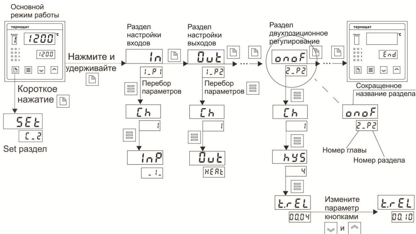
Рисунок 5 – Схема меню
