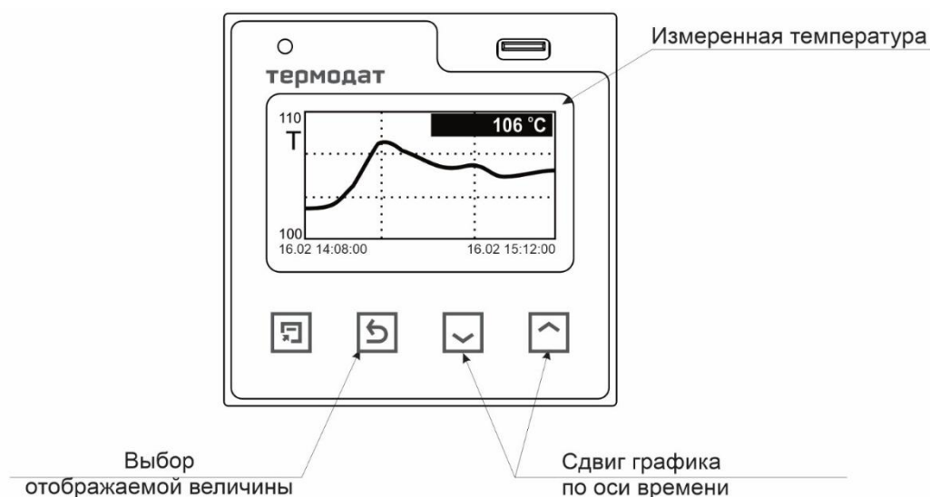
Рисунок 2 – Режим индикации «График»
