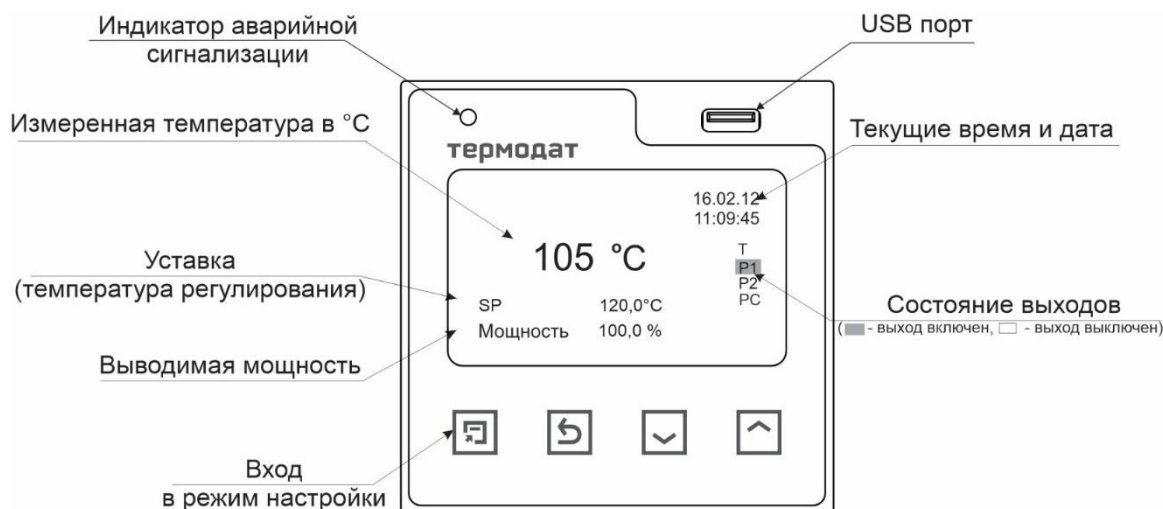
Рисунок 1 – Режим индикации «Текст- значение крупно»
