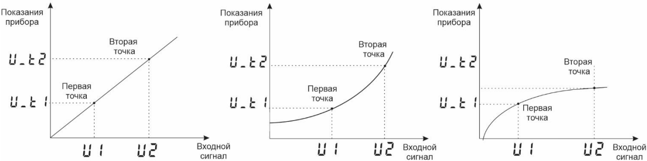
Рисунок 3 –Графики линейной, квадратичной зависимости или зависимости с извлечением квадратного корня для входа
