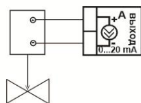
Подключение задвижки с электроприводом
