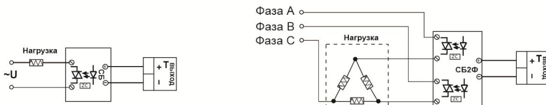
Управление однофазной нагрузкой с помощью блока СБ
