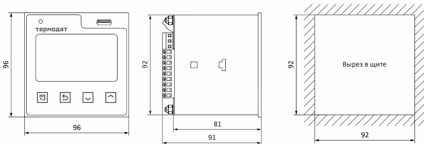
Рисунок 11 – Габаритные размеры прибора Термодат-16К6-A-(F)
