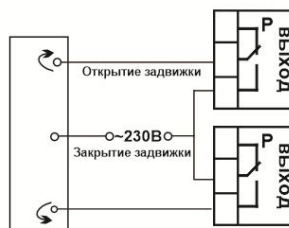
Подключение электрозадвижки
