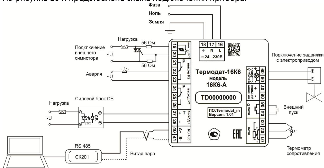
Рисунок 10 – Схема подключения прибора
