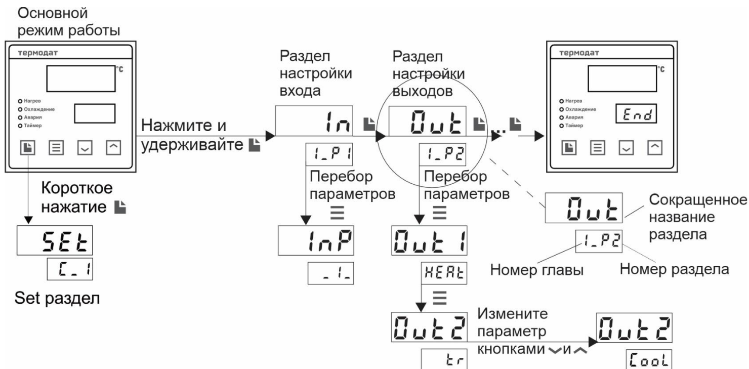
Рисунок 9 – Схема меню
