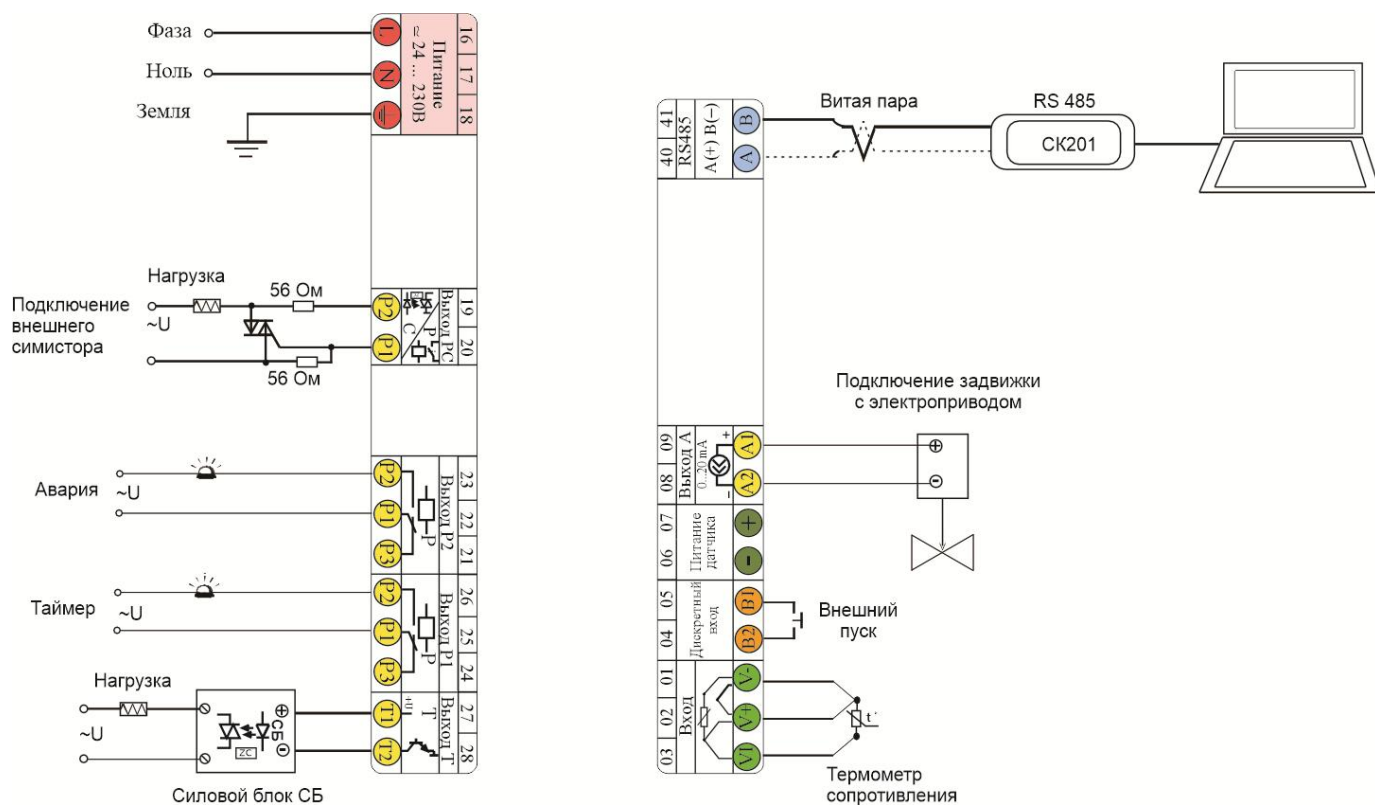
Рисунок 19 – Схема подключения прибора Термодат-12К6-Р6...
