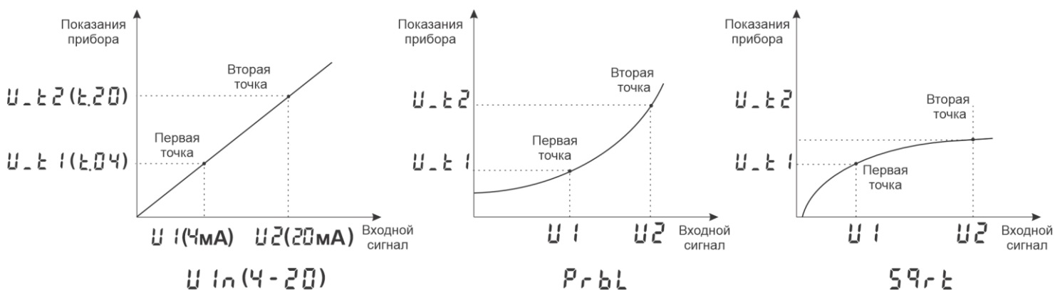
Рисунок 10 – Графики зависимости показаний прибора от входного сигнала при использовании входа типа U.in , PrbL , Sqrt и датчика 4...20
