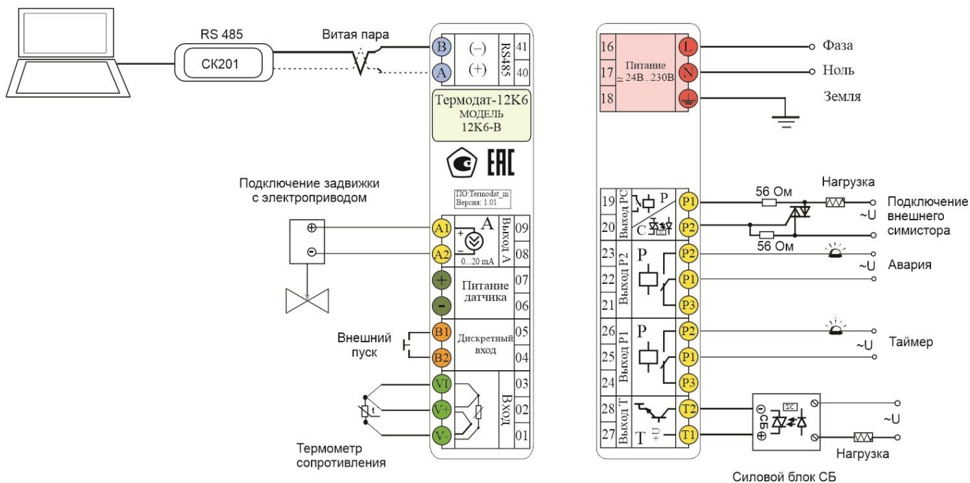
Рисунок 18 – Схема подключения прибора Термодат-12К6-В..., Термодат-12К6-Н...
