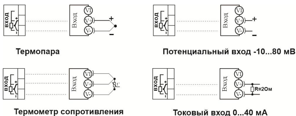
Рисунок 12 – Схемы подключения датчиков
