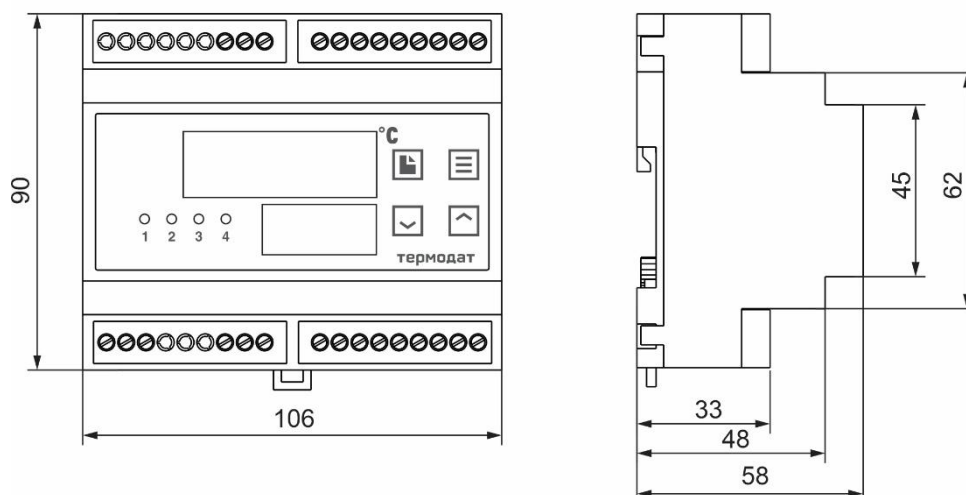
Рисунок 22 – Габаритные размеры прибора Термодат-12К6-P6...
