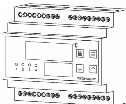
Рисунок 4 – Внешний вид прибора Термодат-12К6-Р6...
