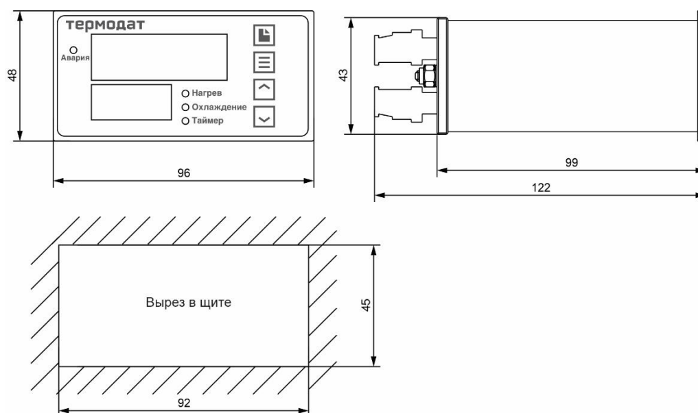
Рисунок 24 – Габаритные размеры прибора Термодат-12К6-Н...
