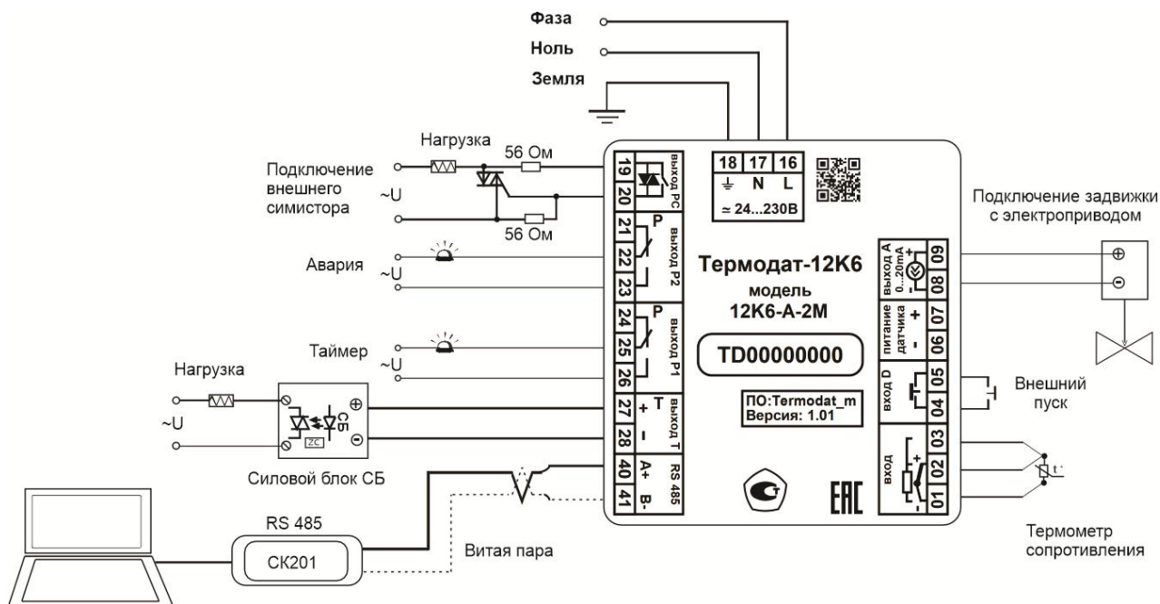
Рисунок 17 – Схема подключения прибора Термодат-12К6-А...
