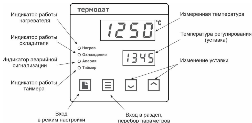
Рисунок 5 – Описание индикаторов и кнопок управления прибора 12К6-А...
