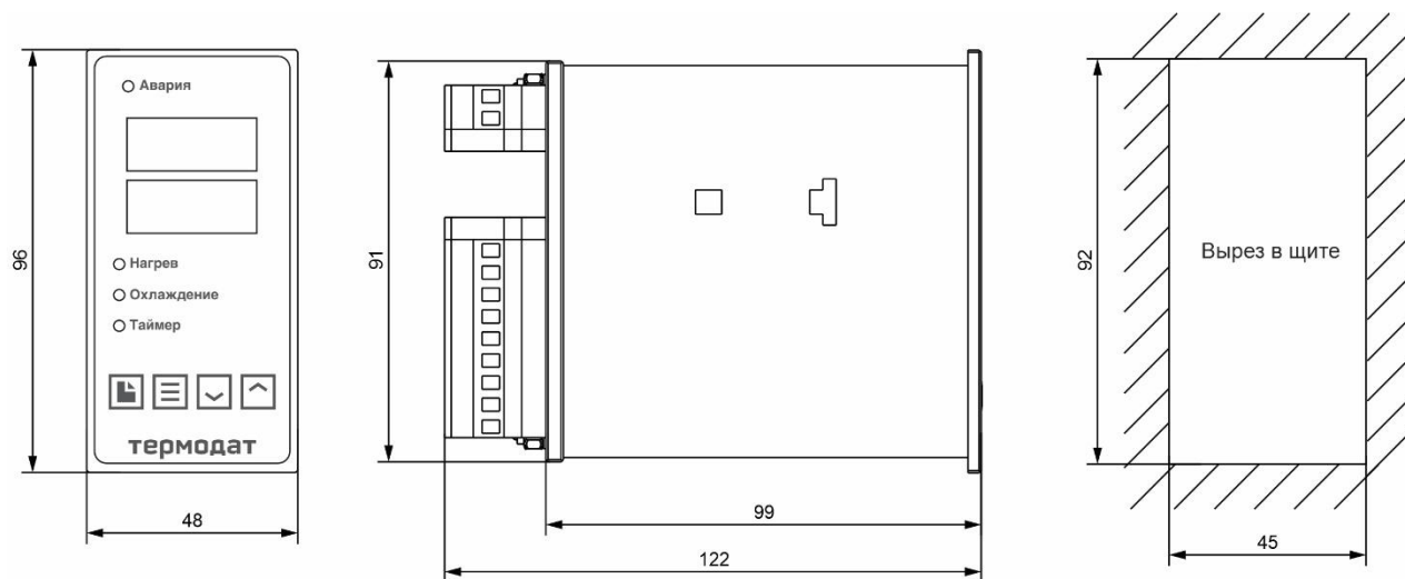
Рисунок 23 – Габаритные размеры прибора Термодат-12К6-В...
