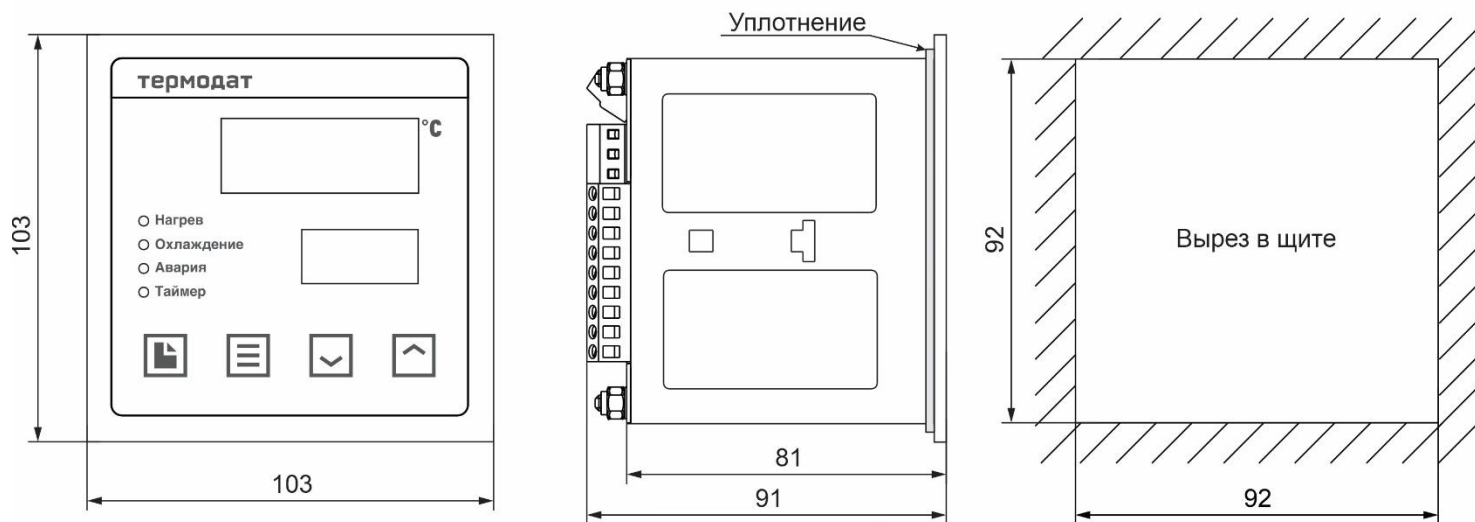
Рисунок 21 – Габаритные размеры прибора Термодат-12К6-A7...
