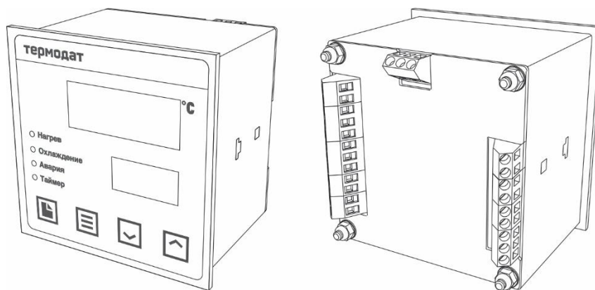
Рисунок 1 – Внешний вид прибора Термодат-12К6-А...
