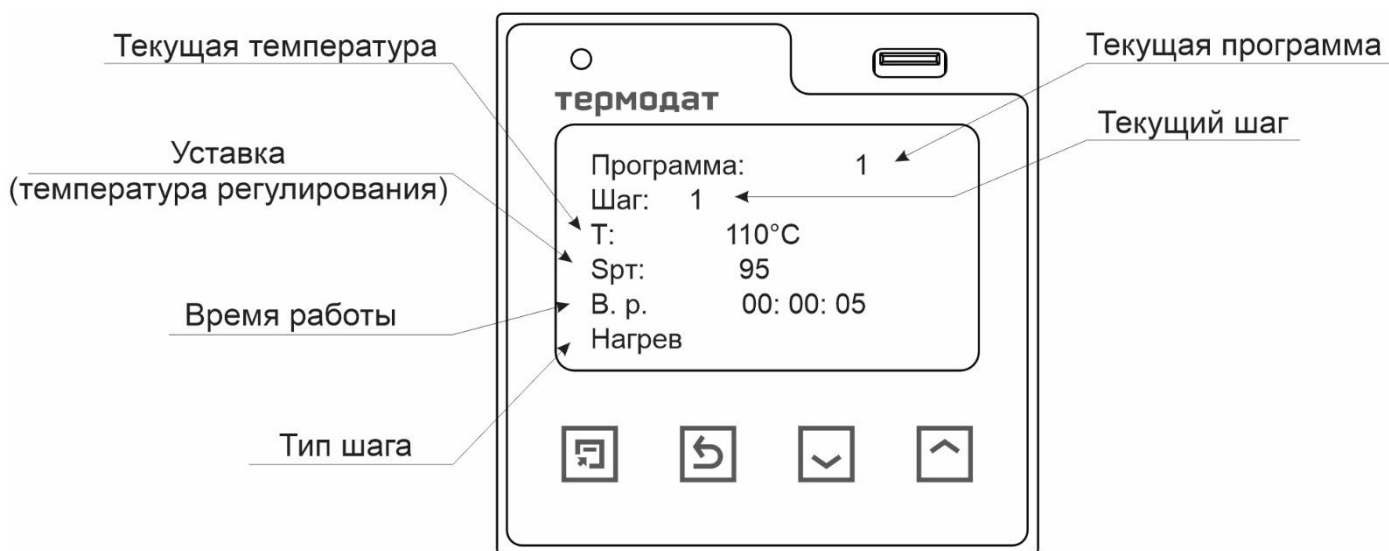
Рисунок 4 - Режим индикации «Текст- состояние программы»
