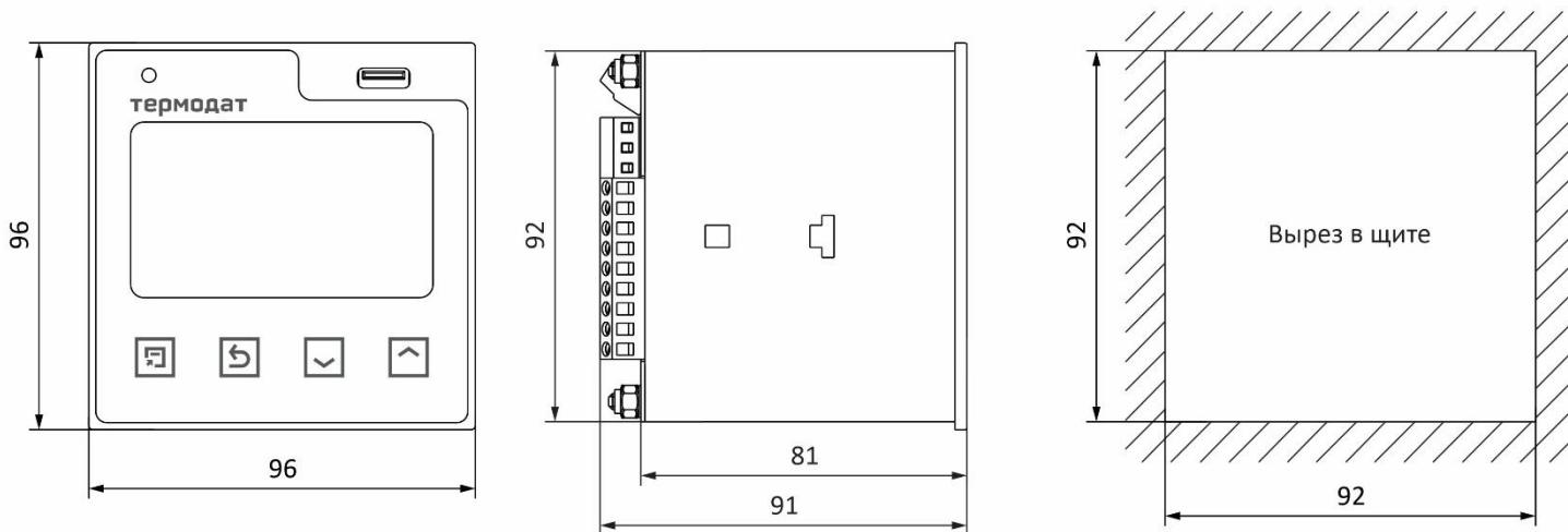
Рисунок 16 – Габаритные размеры прибора Термодат-16Е6-А-(F)-(Eth)
