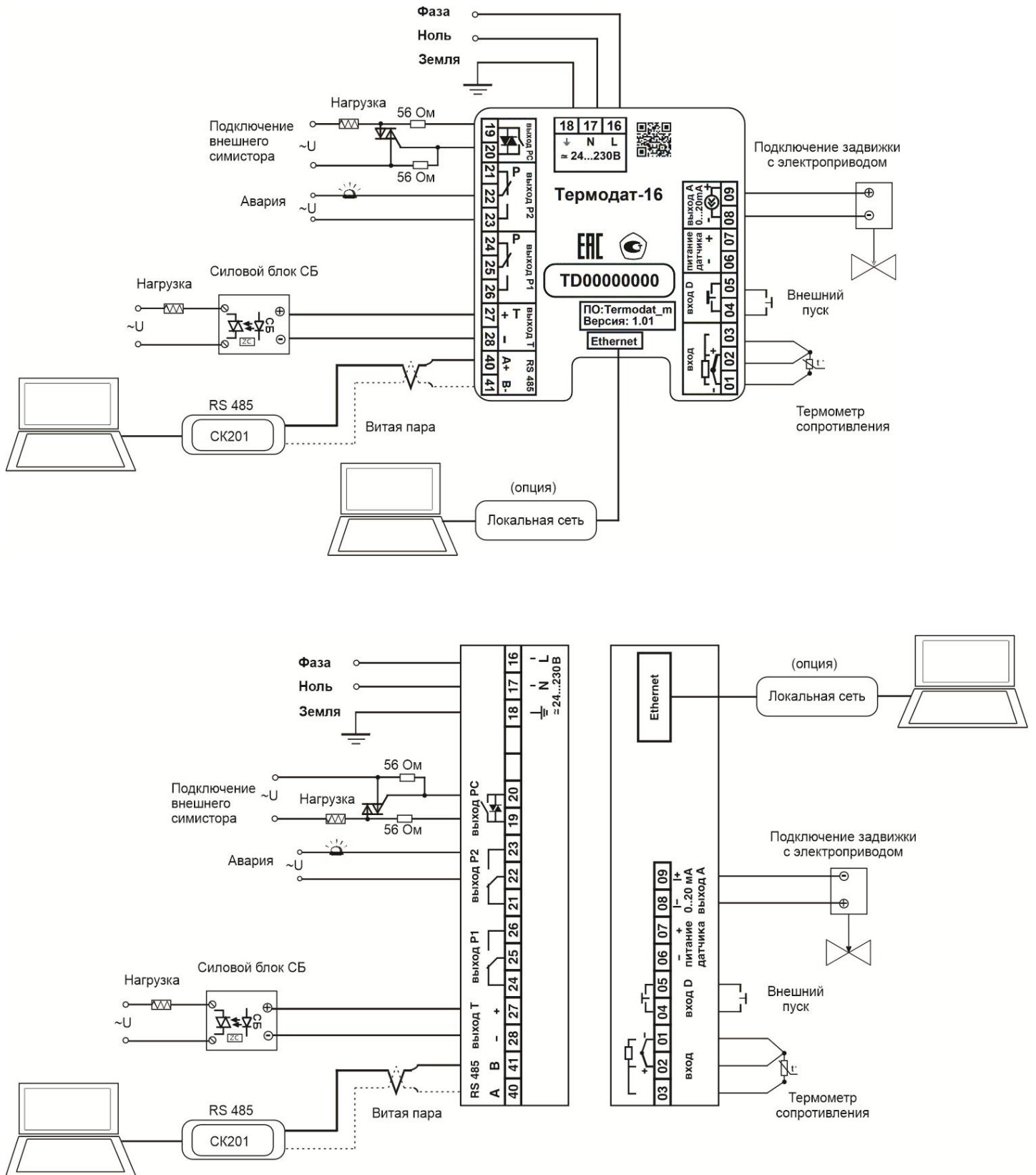
Рисунок 14 – Схема подключения прибора
