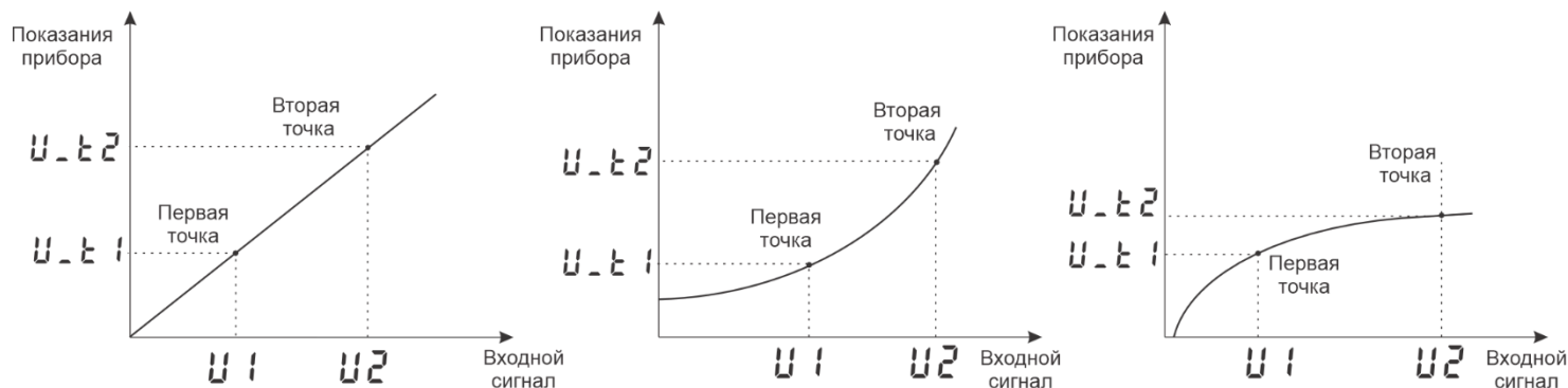
Рисунок 7 – Графики линейной, квадратичной зависимости или зависимости с извлечением квадратного корня для входа
