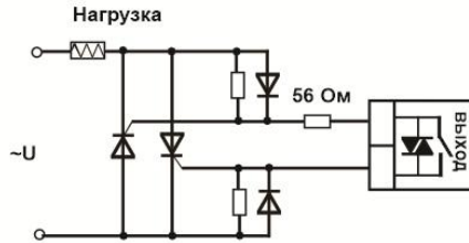
Подключение внешних тиристорov
