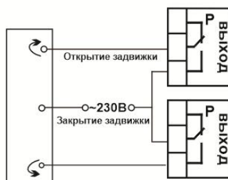
Подключение электрозадвижки
