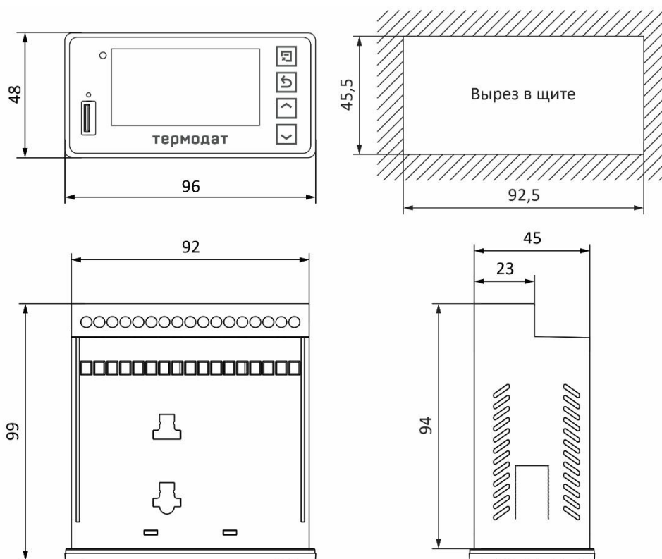
Рисунок 15 – Габаритные размеры прибора Термодат-16Е6-Н-(F)-(Eth)
