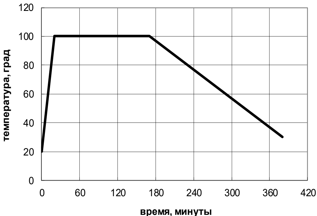
Рисунок 6 – График режима термообработки
