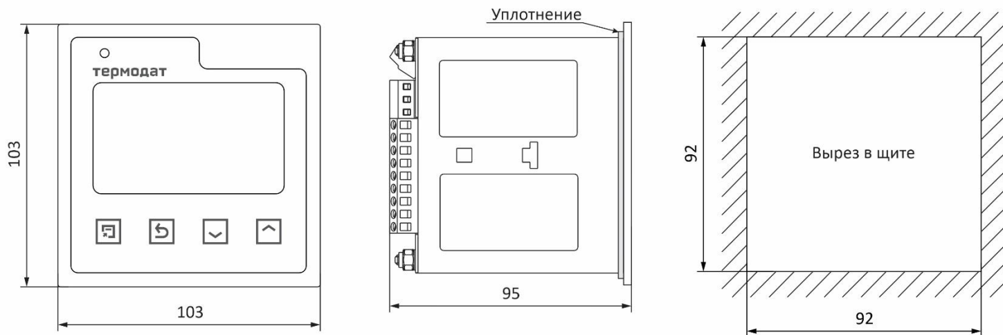
Рисунок 17 – Габаритные размеры прибора Термодат-16Е6-А7
