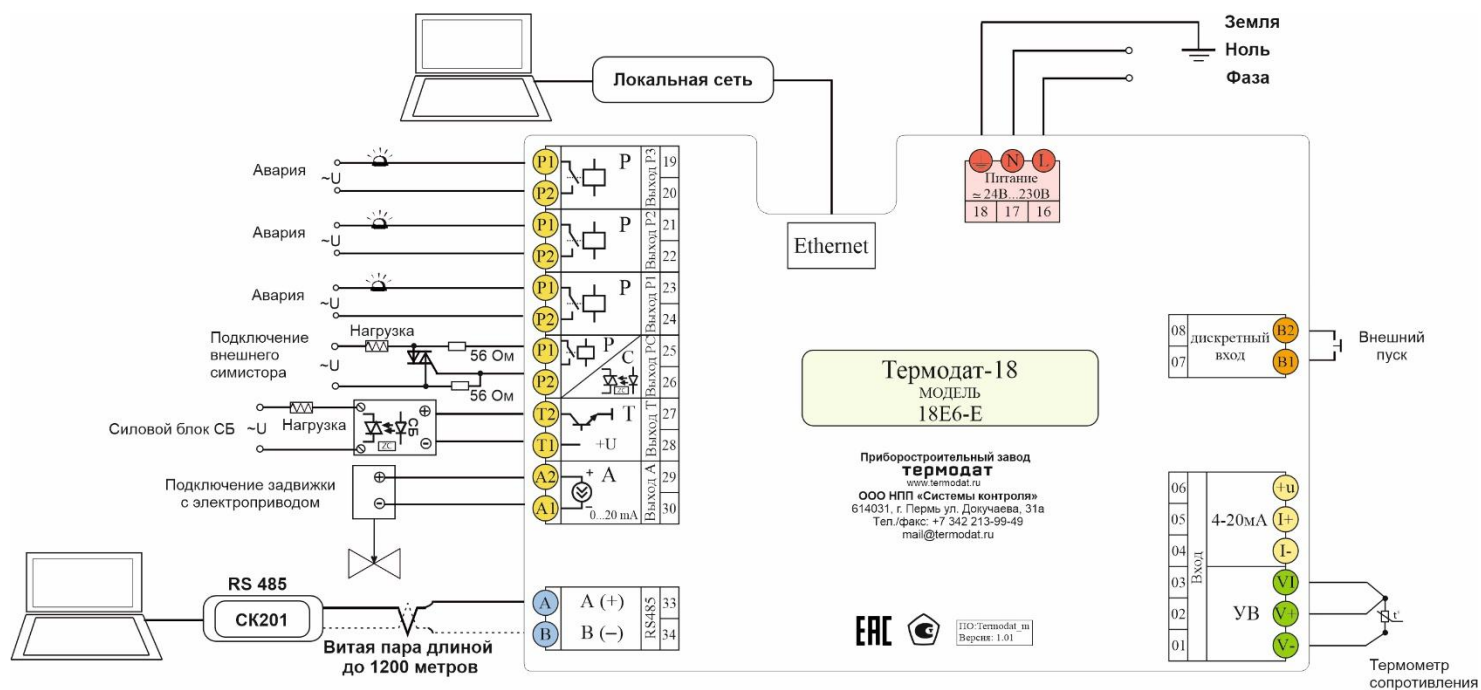
Рисунок 5 - Схема подключения прибора
