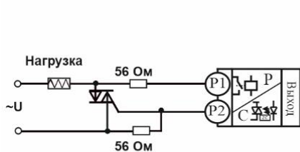
Подключение внешнего симистора
