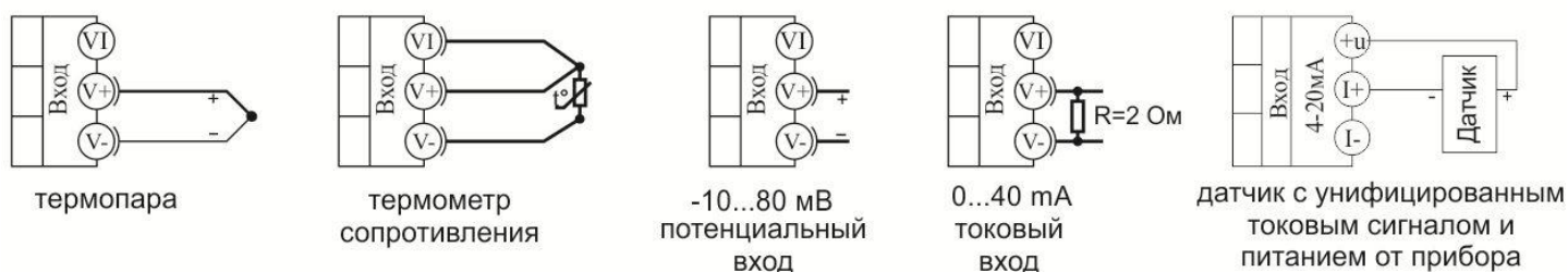
Рисунок 1 - Схемы подключения датчиков
