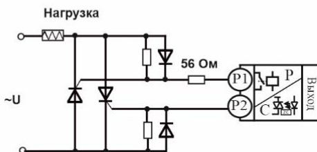
Подключение внешних тириستоров
