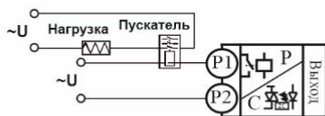
Подключение нагрузки мощностью более 2,3 кВт с помощью электромагнитного пускателя
