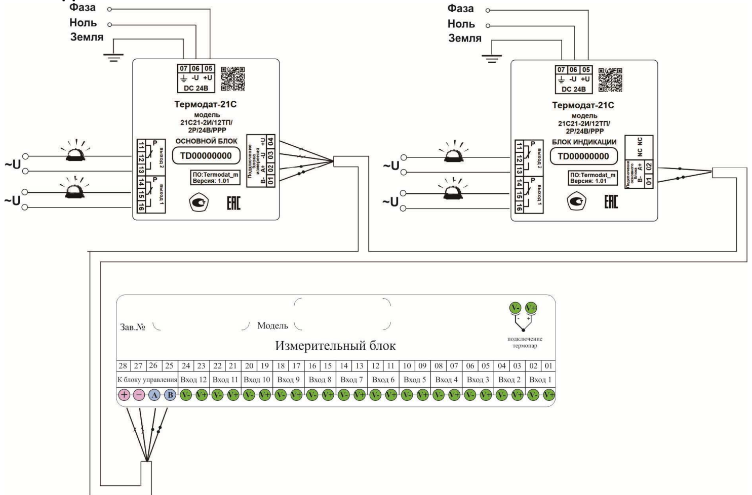
Рисунок 5 – Схема подключения прибора 21С21-2И-12ТП/2Р/24В/РРР
