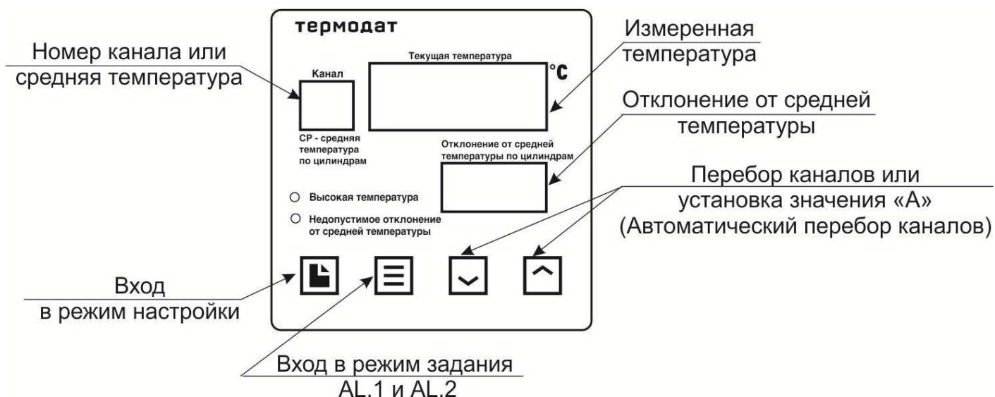
Рисунок 1 – Внешний вид прибора в основном режиме работы
