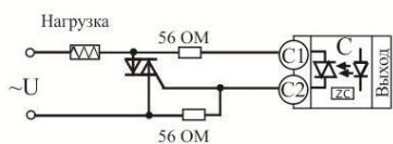
Подключение внешнего симистора
