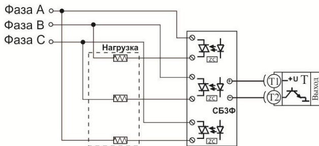
Подключение трехфазной нагрузки в шестипроводной схеме
