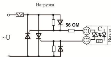
Подключение внешних тиристор
